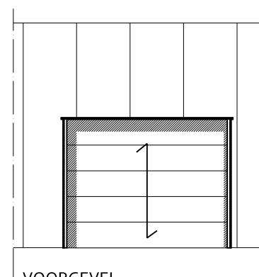
- VOORGEVEL -
