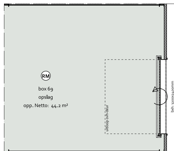
- PLATTEGROND -
